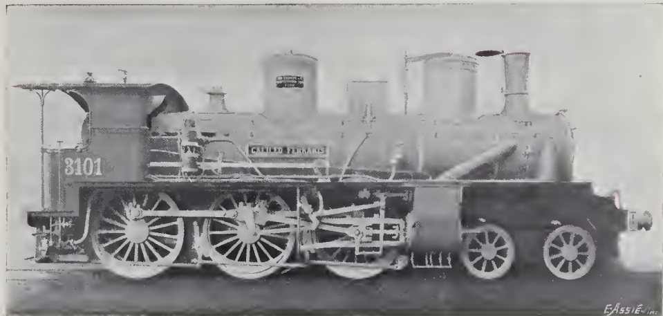
« GALILEO FERRARIS » LOCOMOTIVA DELLA CASA G. ANSALDO E C.
